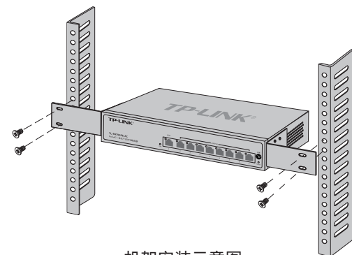
机架安装示意图
