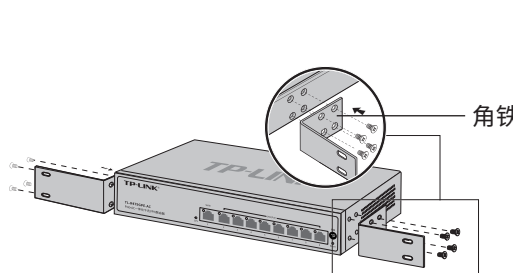
角铁安装示意图
